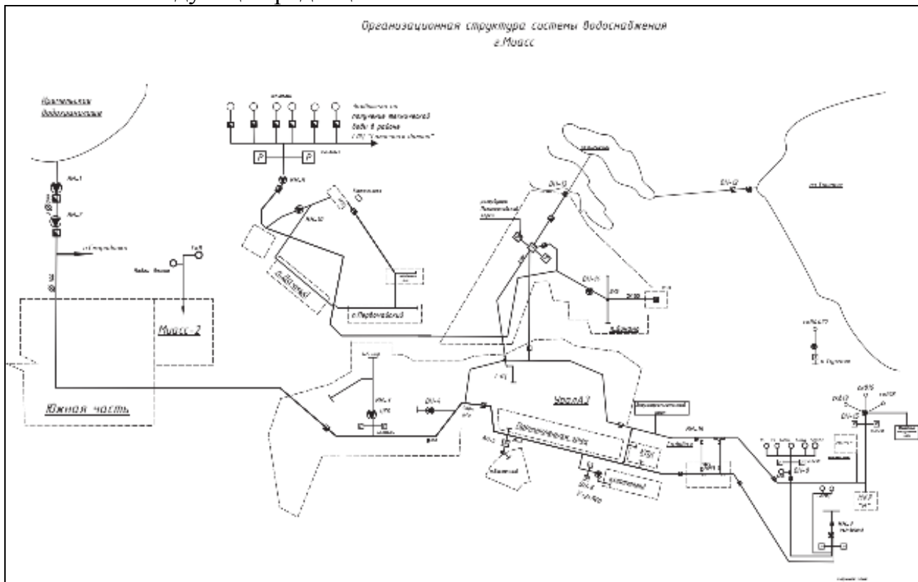
рис. 2.1.4.2.1. Технологическая схема системы водоснабжения ОАО «Миассводоканал» г. Миасс.
